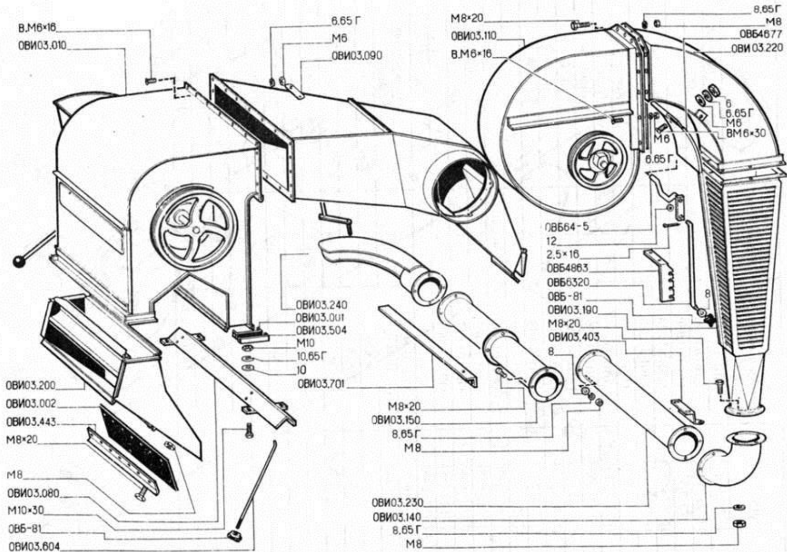
Рис. 15. Часть воздушная ОВИ 03.000.
